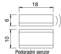
Podgradni senzor
