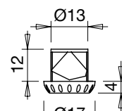
Ugradni senzor
