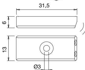
Ugradni senzor 20°
