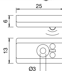
Ugradni senzor 90°
