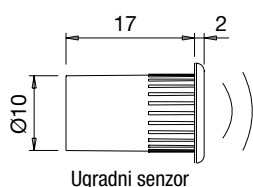
Ugradni senzor
