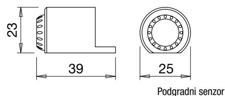
Podgradni senzor
