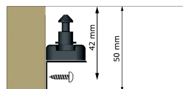
Skica pokazuje deo za zatvaranje sa bravicom
