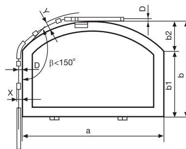
GEZE OL 90 N Flachbogenfenster mit 1 Schere
