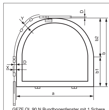
GEZE OL 90 N Rundbogenfenster mit 1 Schere
