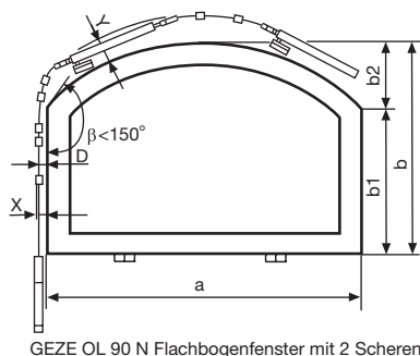
GEZE OL 90 N Flachbogenfenster mit 2 Scheren
