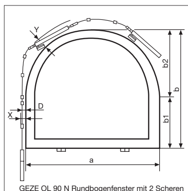
GEZE OL 90 N Rundbogenfenster mit 2 Scheren
