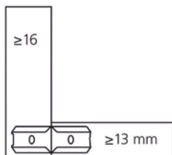
Različiti ugaoni spojevi od 30°-180°
