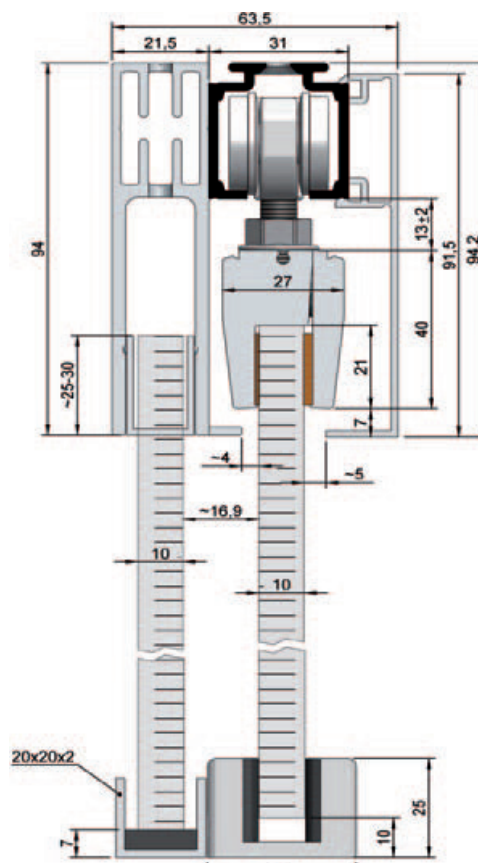
sa bočnim profilom
